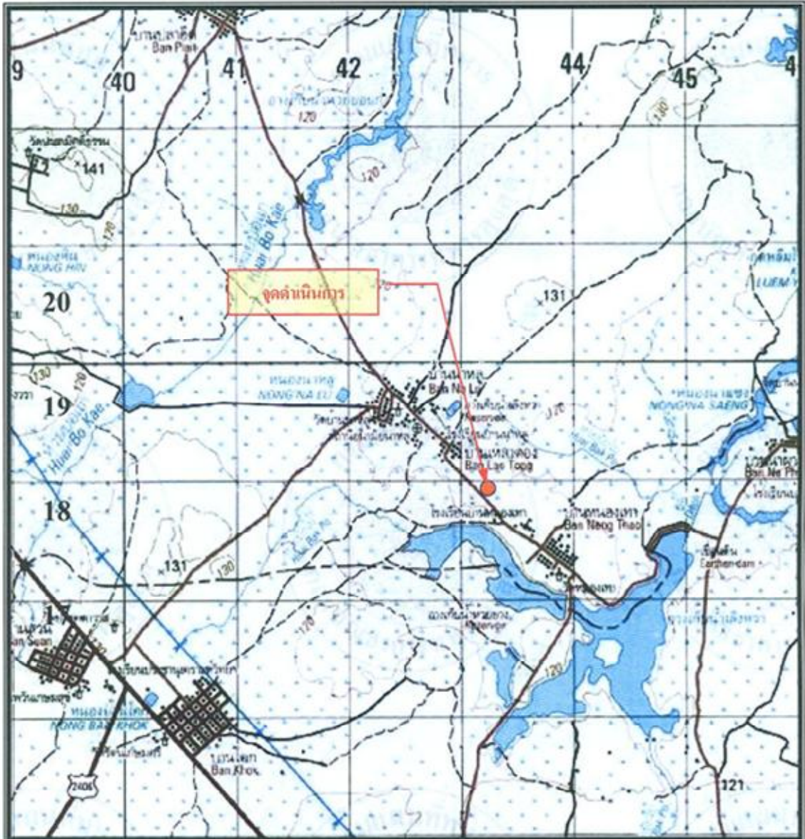
โครงการปรับปรุงอ่างเก็บน้ำห้วยยาง บ้านหนองเทา ตำบลนาแก อำเภอคำชะอี จังหวัดยโสธร พิกัด UTM 443362E - 1718360N ระวัง 5840 II ตามแผนที่มาตราส่วน 1: 50,000 ของกรมแผนที่ทหาร ลำดับชุด L 7018
